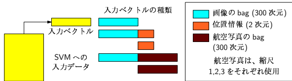
図 5 キーワードごとの SVM への入力ベクトル
