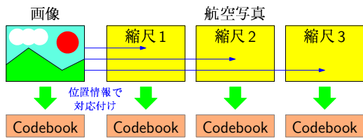
図 4 Codebook の生成
