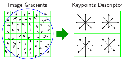
図 1 SIFT 特徴
