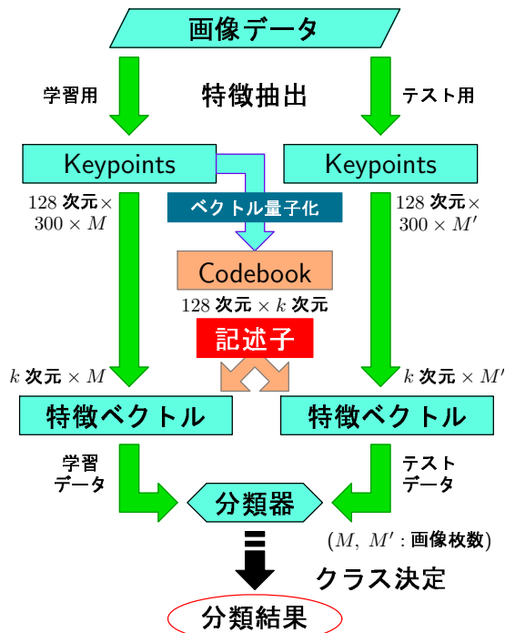
図 2 Bag of Keypoints 手法
